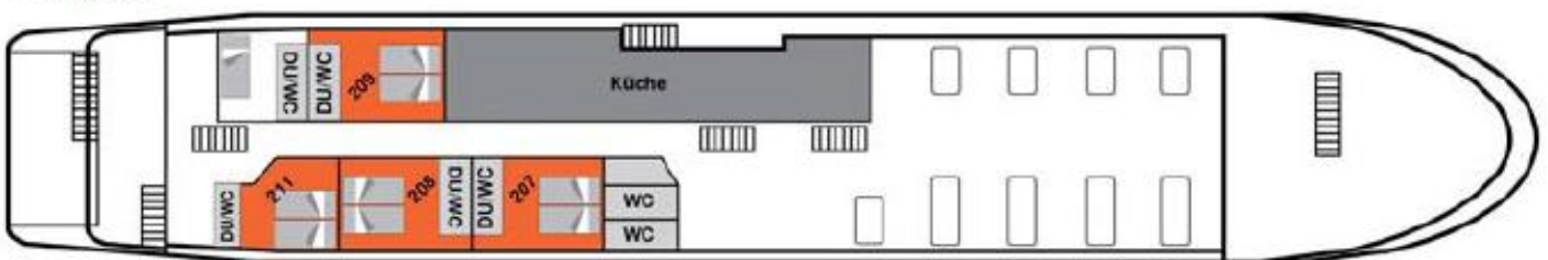
Hauptdeck
